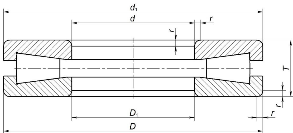
Рисунок 1 – Конструктивное исполнение 01
