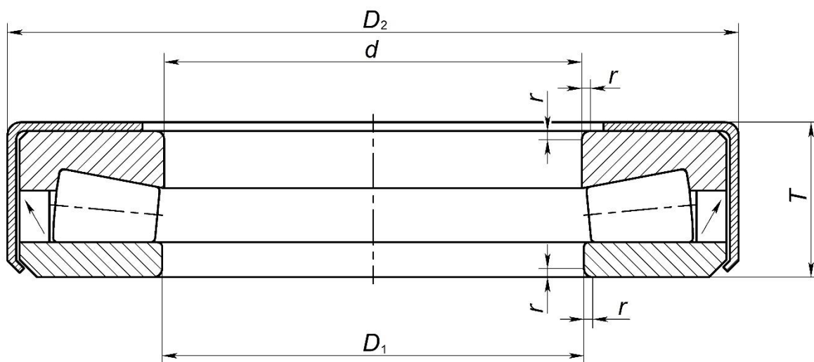
Рисунок 1 – Конструктивное исполнение 01
