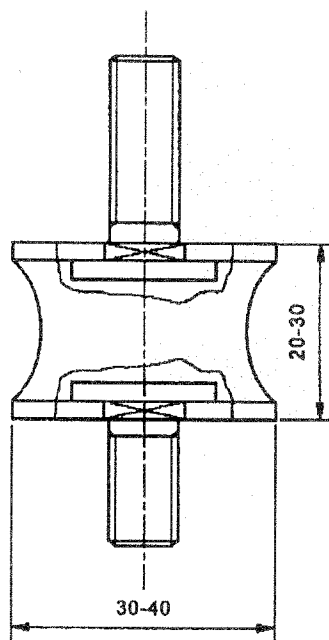
Рисунок 4 – Типичная резиновая втулка для крепления испытательной стенки
