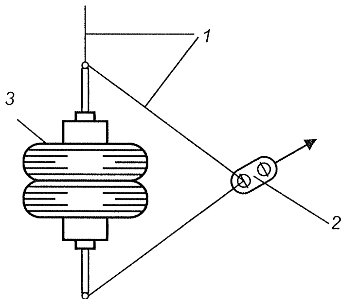
Рисунок Ж.1 – Пример устройства для создания динамических нагрузок
