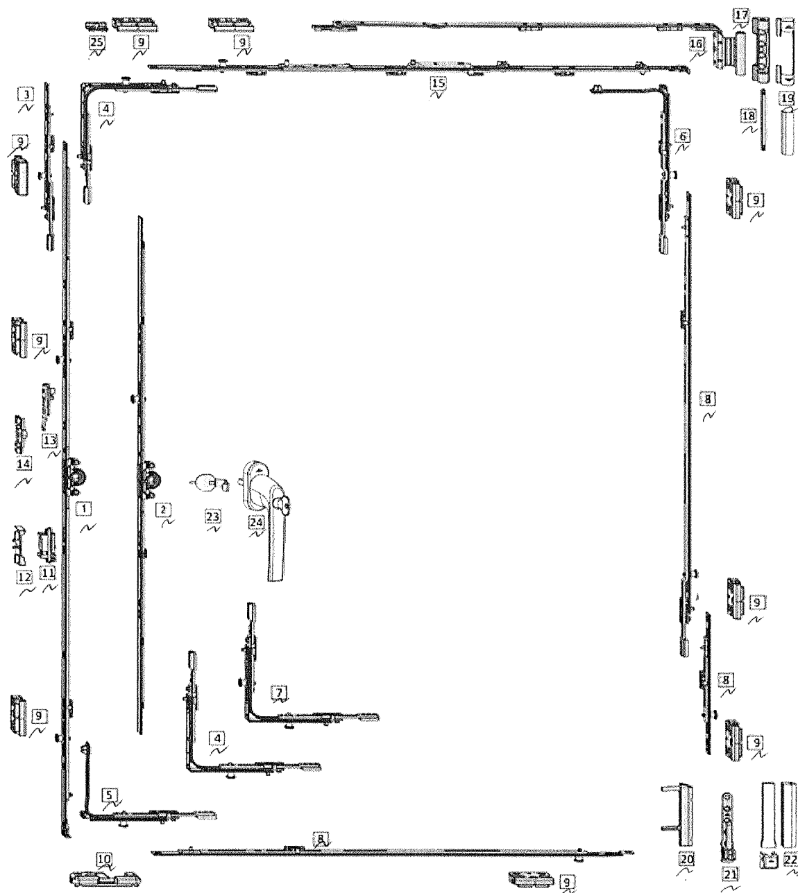
Рисунок И.1 – Пример комплекта противовзломного устройства защитного окна
