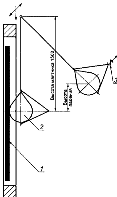
Рисунок Ж.1 – Пример устройства для создания динамических нагрузок
