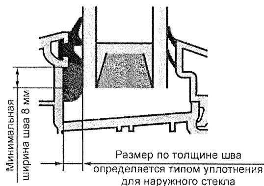
Рисунок 2 – Пример конструкции узла клейки стеклопакета
