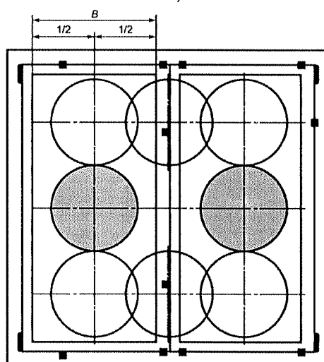
Рисунок Г.1 – Точки приложения динамических нагрузок на одностворчатом оконном (дверном балконном) блоке
