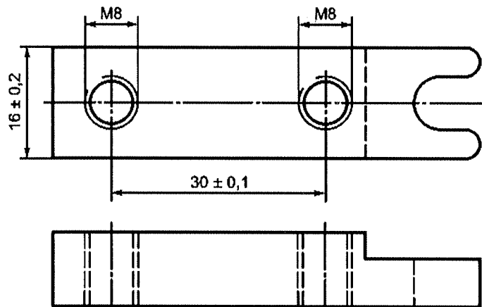
Рисунок Д.2 – Пример специальной стальной пластины (адаптера-переходника) для передачи статической нагрузки на запирающие элементы
