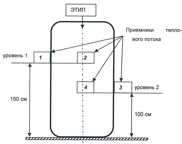
Рисунок 1 - Схема расположения приемников теплового потока
