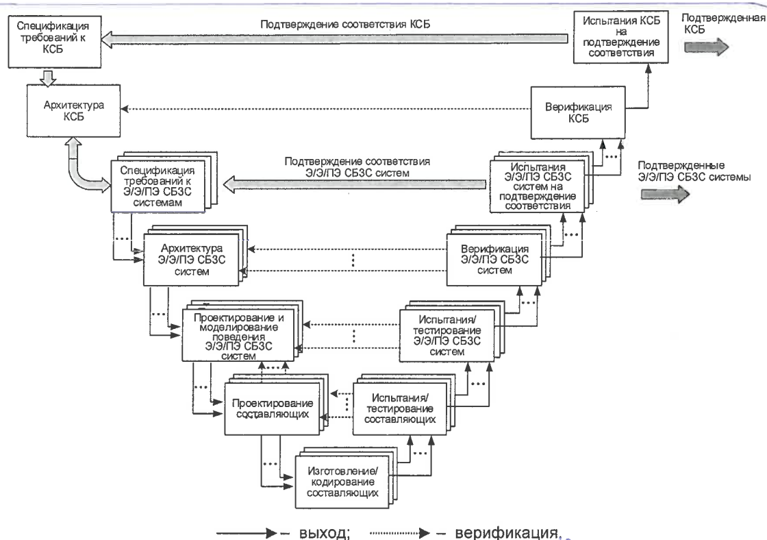
Рисунок 6 — V-образная модель стадий проектирования и реализации КСБ
