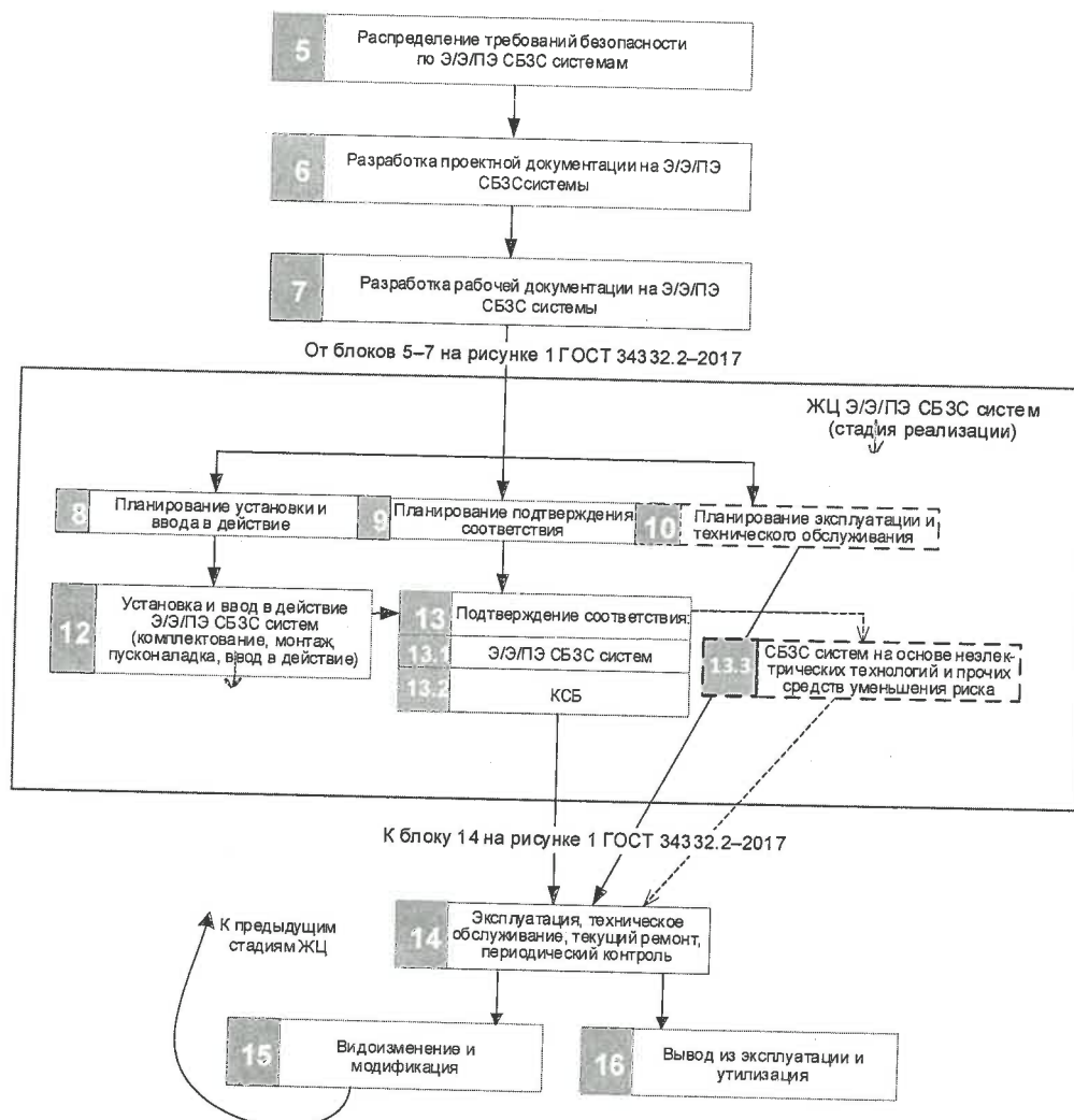
Рисунок 5 — Структура ЖЦ Э/Э/ПЭ СБЗС системы (стадии проектирования и реализации)
