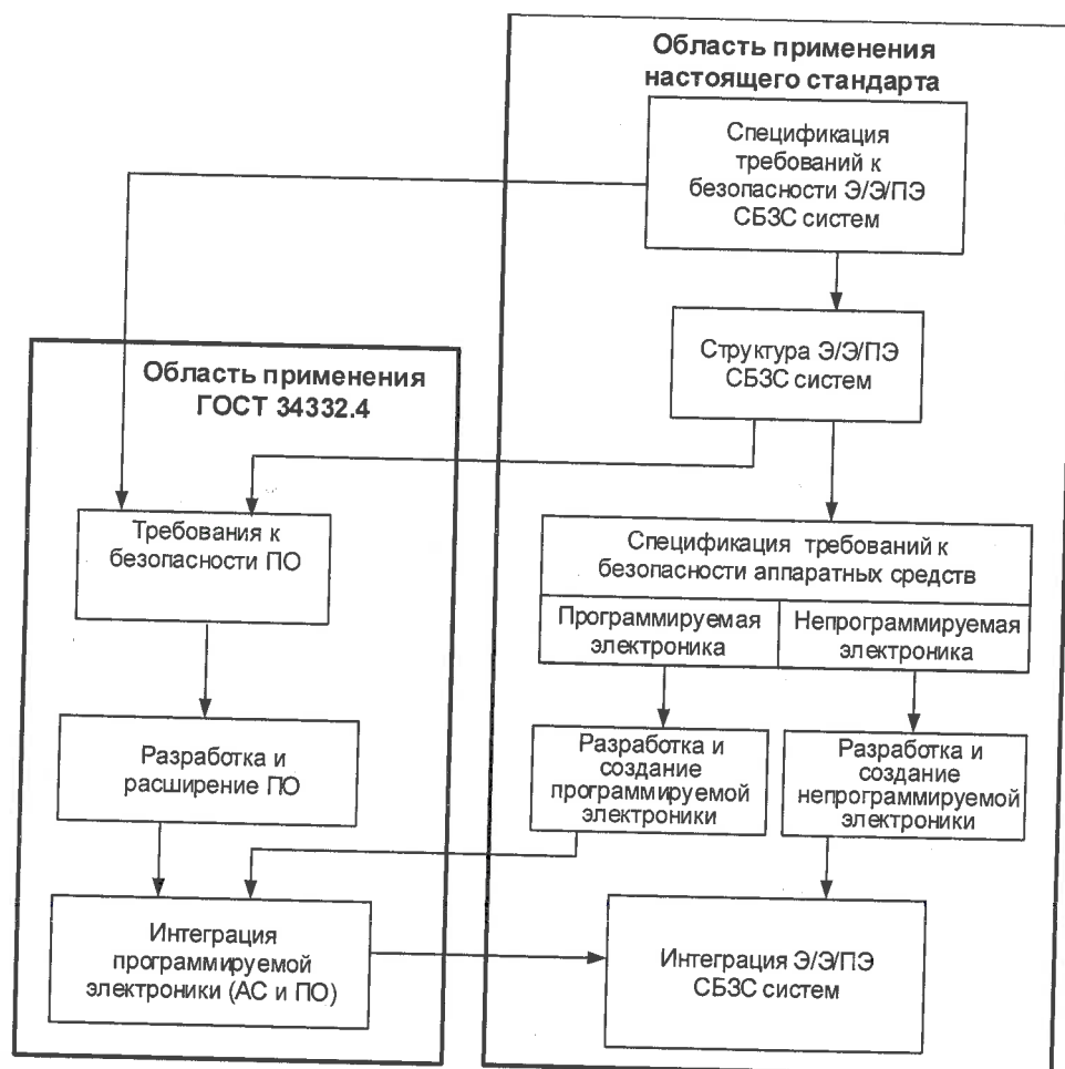
Рисунок 2 — Взаимосвязь областей применения настоящего стандарта и ГОСТ 34332.4
