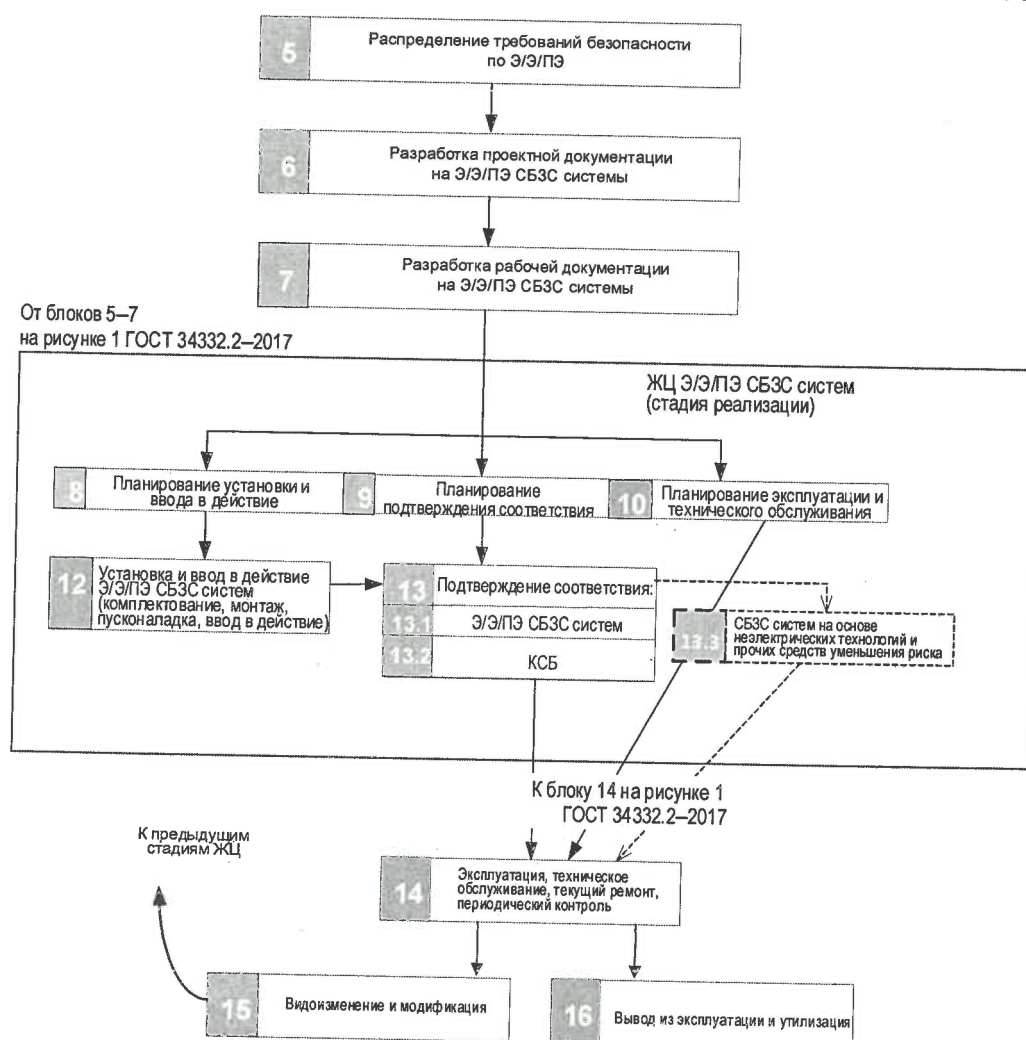
Рисунок 4 — Часть ЖЦ ПО ПЭ СБЗС системы
