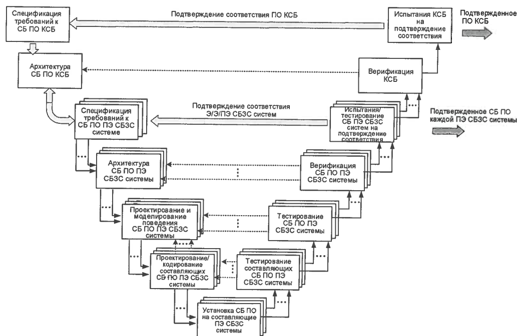
Рисунок 6 — V-образная модель стадий разработки и реализации ЖЦ СБ ПО КСБ
