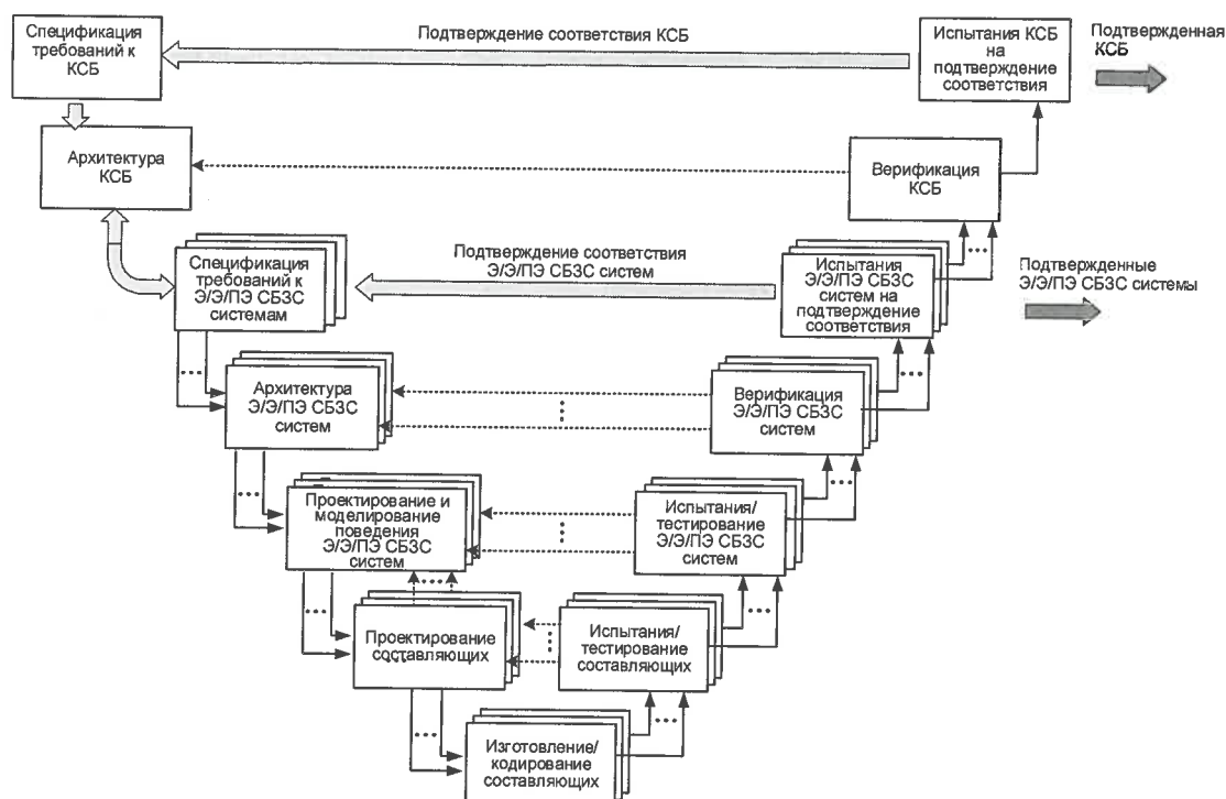
Рисунок 5 — V-образная модель стадий разработки и реализации ЖЦ КСБ
