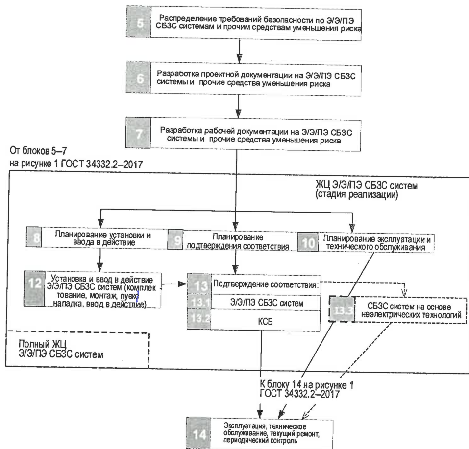
Рисунок 3 — Часть ЖЦ Э/Э/ПЭ СБЗС системы
