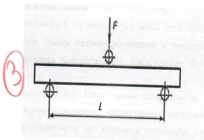
Рисунок И.1 - Схема испытания на предел прочности при изгибе
