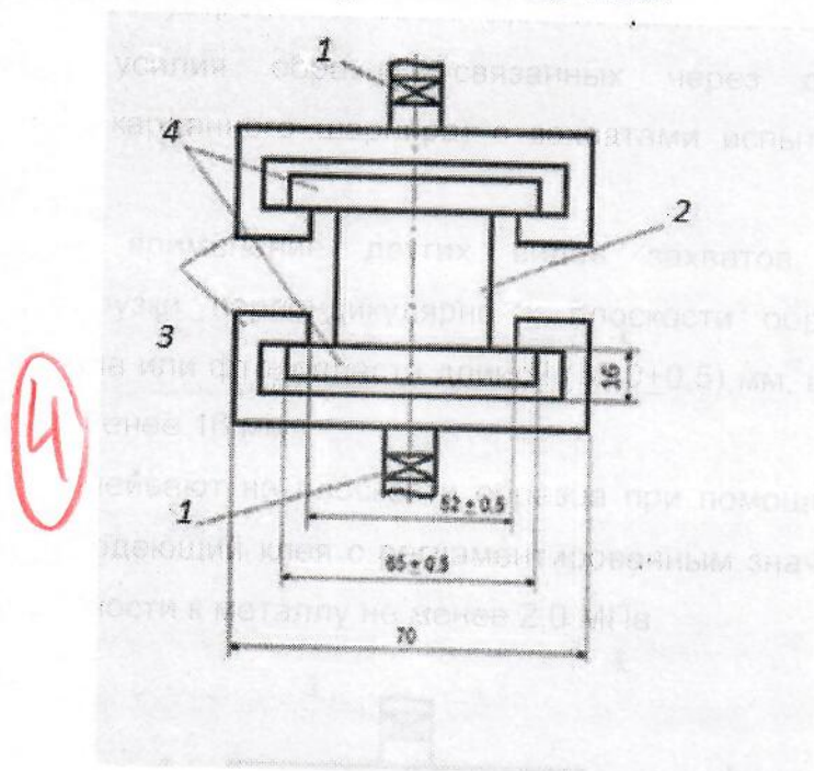
Рисунок К.1 - Испытательная машина
