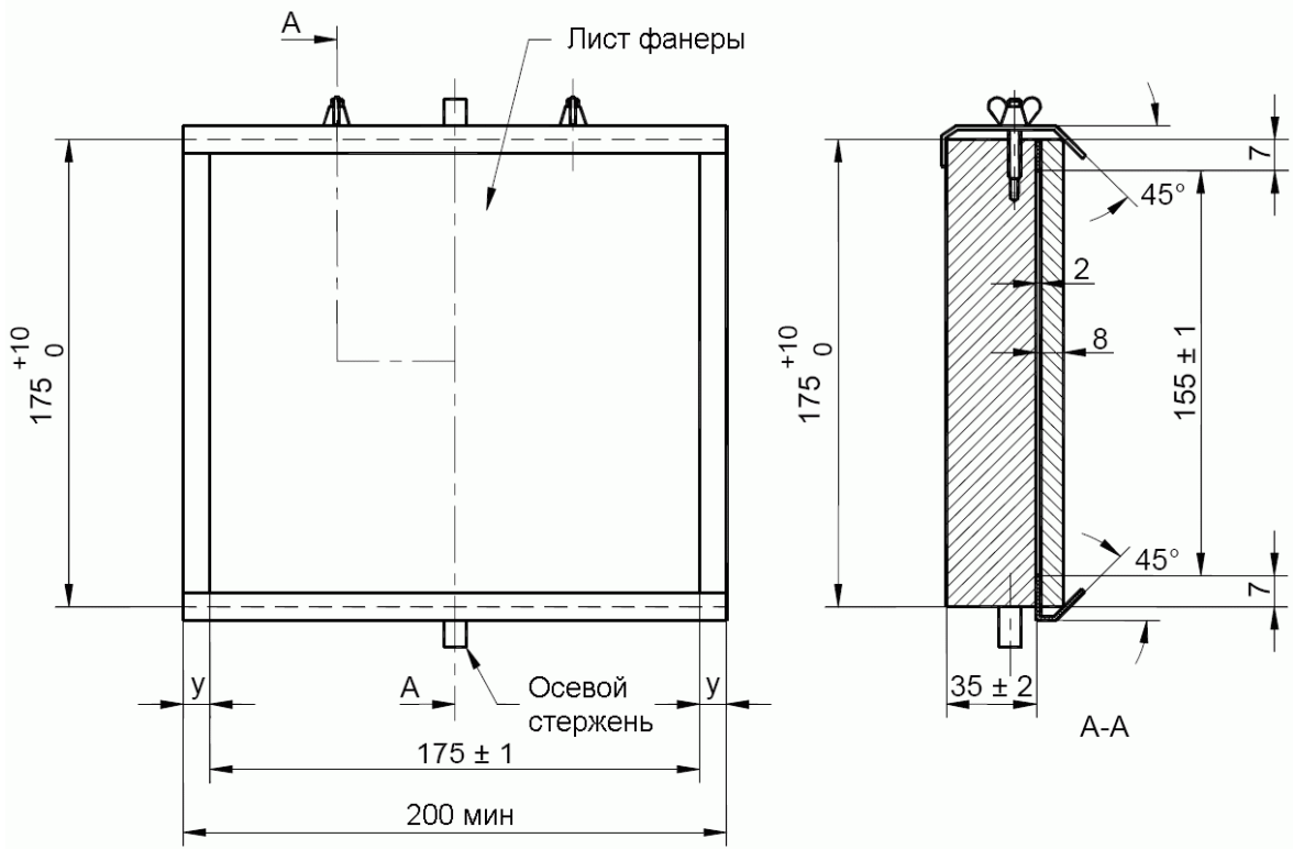
Рисунок D.2 — Крепежное приспособление
