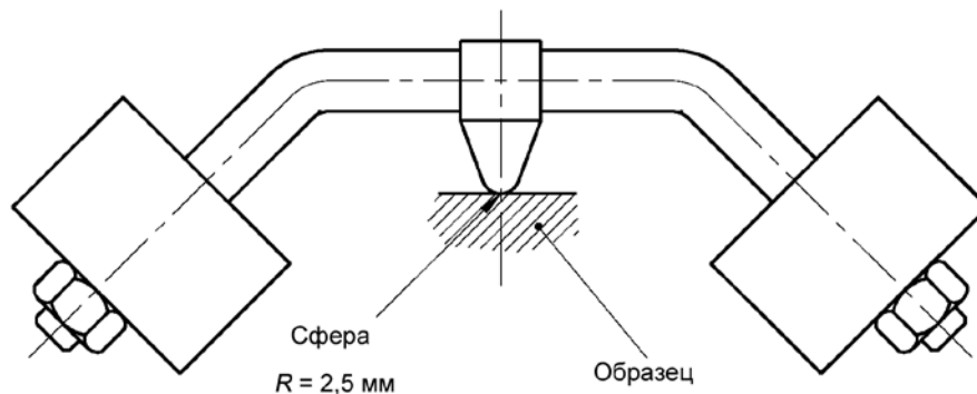
Рисунок 1 — Устройство для испытаний вдавливанием шарика
