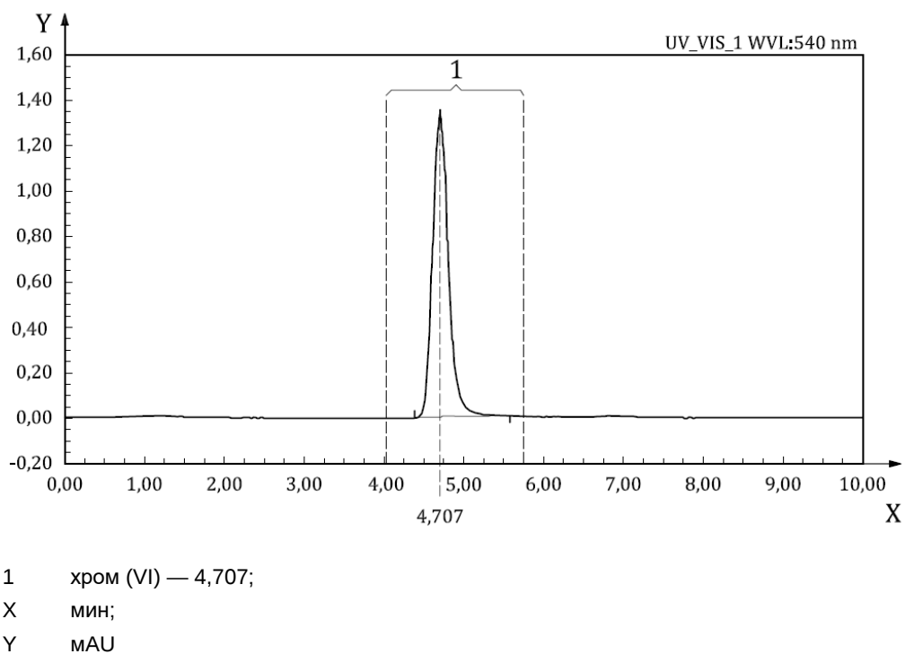
Рисунок С.3 — Хроматограмма образца натуральной кожи концентрацией 3 мг/кг
