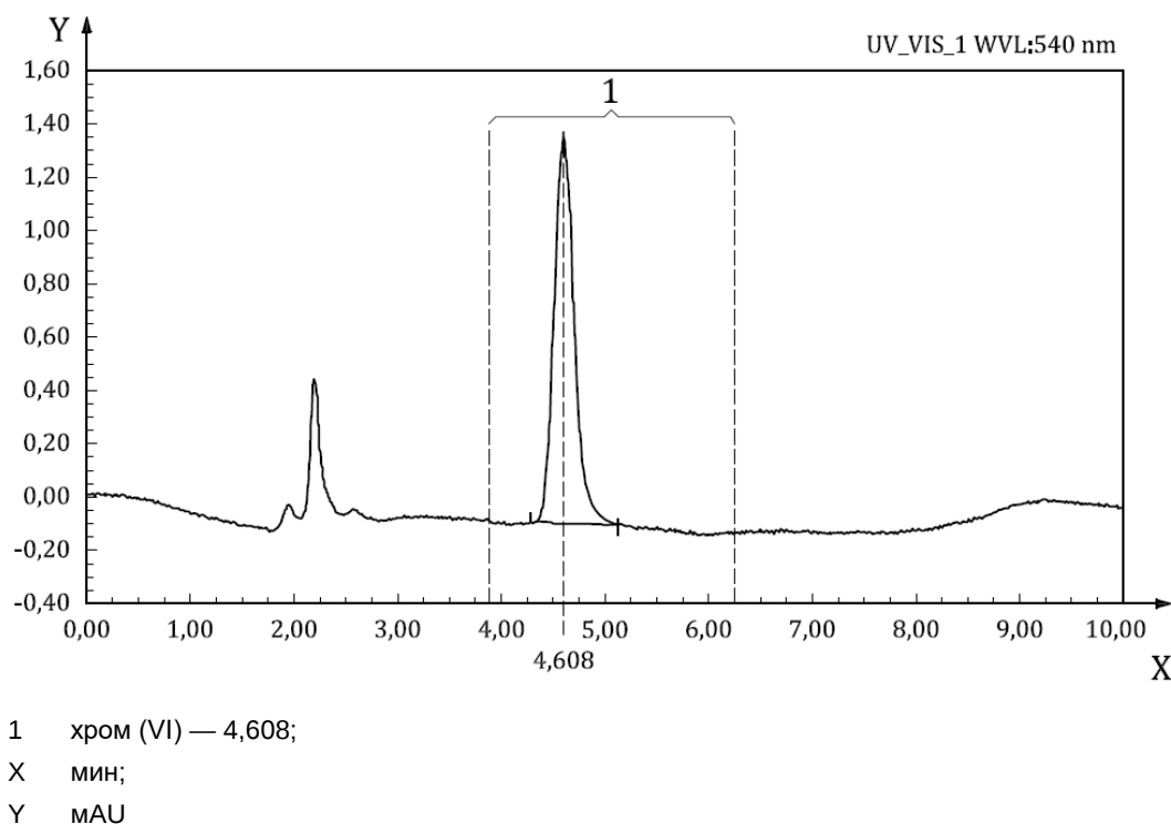
Рисунок С.2 — Хроматограмма стандартного раствора концентрацией 5 мкг/л (соответствует первому уровню калибровочной кривой)
