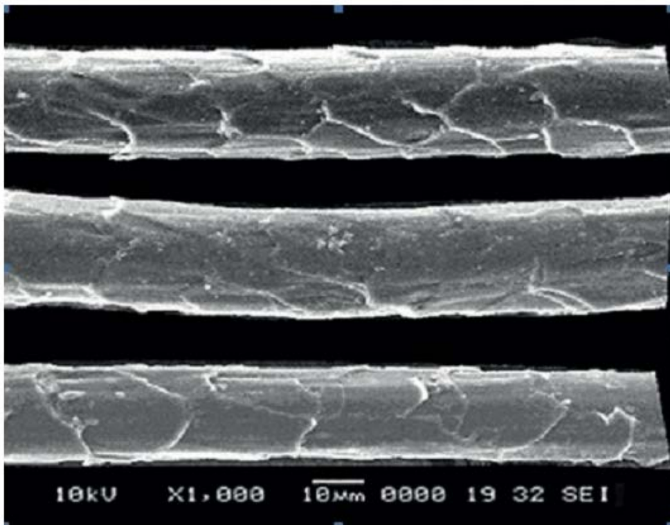
Рисунок В.59 — Изображение волокон с «размытыми» чешуйками
