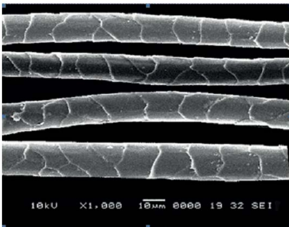
Рисунок В.43 — Изображение волокон с плохим блеском
