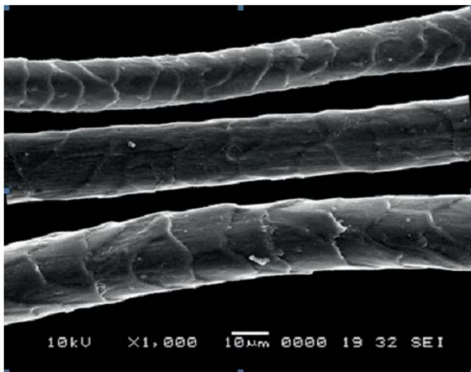
Рисунок В.64 — Изображение волокон безусадочной шерсти
