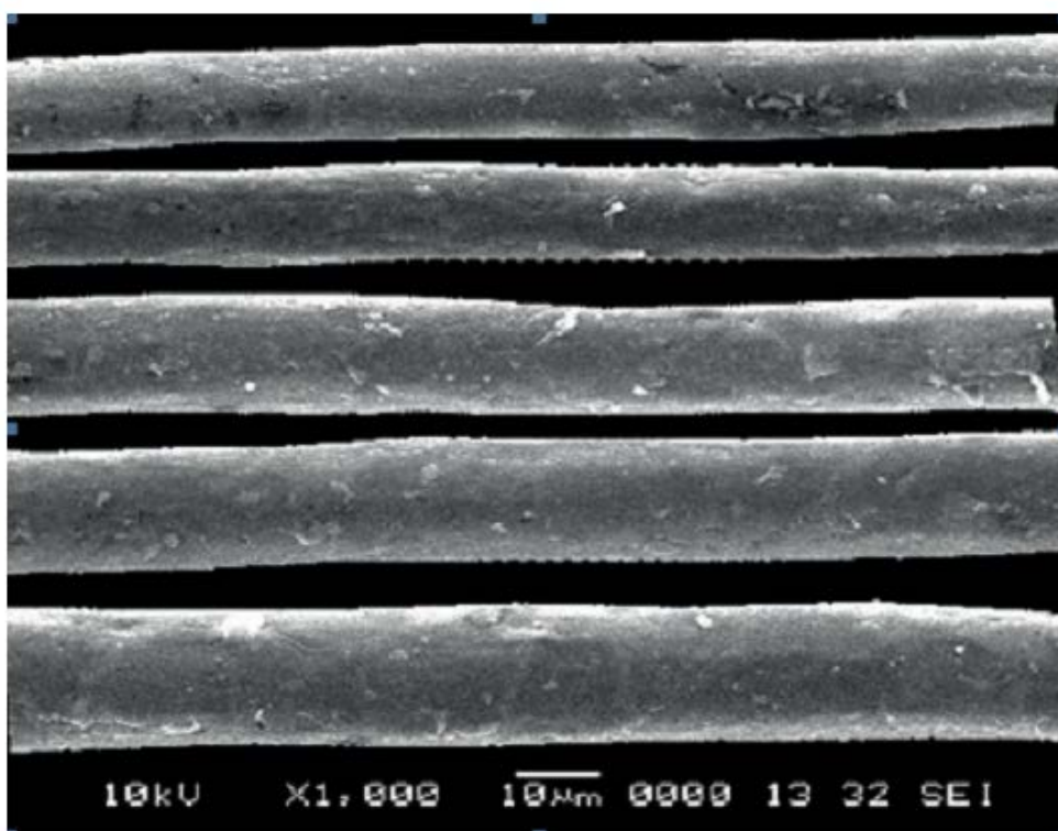
Рисунок В.65 — Изображение волокон мерсеризованной шерсти
