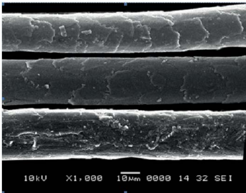
Рисунок В.40 — Изображение волокон с поврежденными чешуйками
