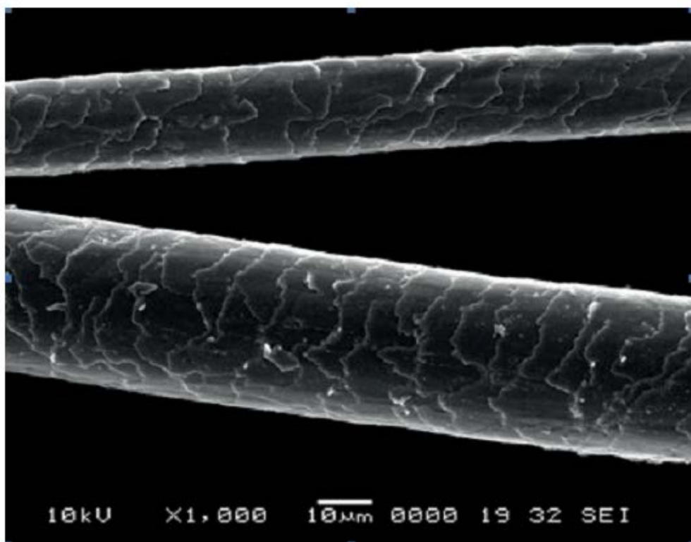
Рисунок В.75 — Изображение волокон шерсти альпаки
