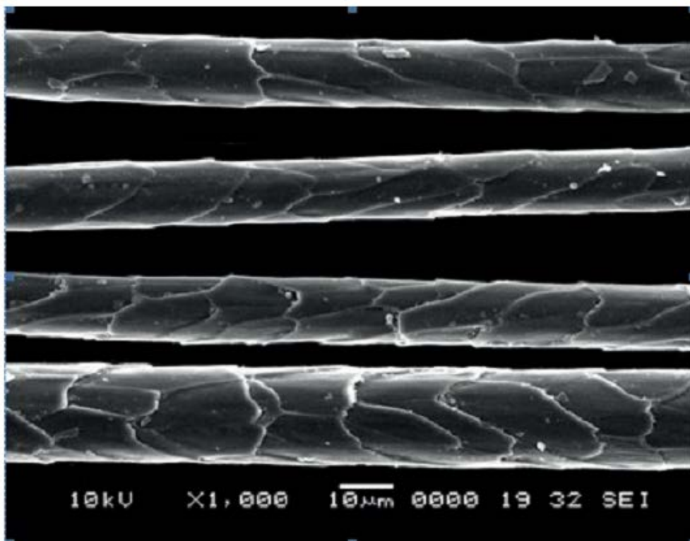
Рисунок В.67 — Изображение типичных волокон верблюжьей шерсти
