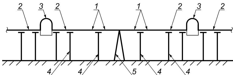
1 — средний пролет; 2 — крайний пролет; 3 — компенсатор; 4 — подвижная опора; 5 — неподвижная опора
