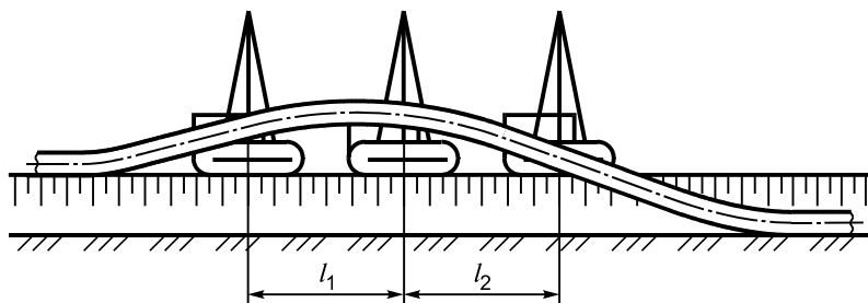
Рисунок А.2 — Схема расстановки трубоукладчиков при непрерывной укладке плети газопровода свыше DN\ 700 до DN\ 900 включительно
