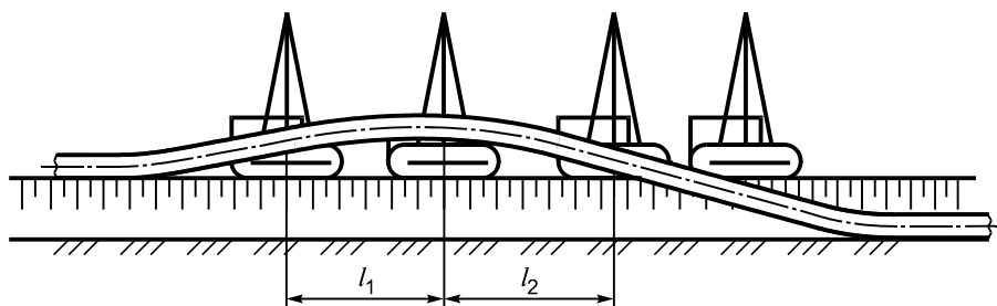
Рисунок А.2 — Схема расстановки трубоукладчиков при непрерывной укладке плети газопровода свыше DN\ 700 до DN\ 900 включительно
