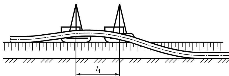
l_1 — расстояние между трубоукладчиками
