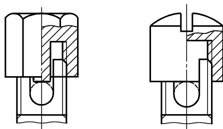
Рисунок 14g — Закрытые винтовые выводы с прижимной гайкой
