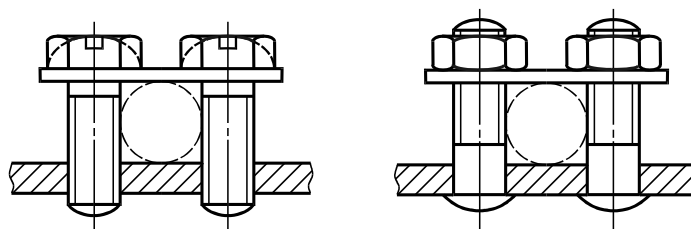
Рисунок 14е — Пластичатые выводы
