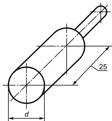
Материал щупов — сталь
