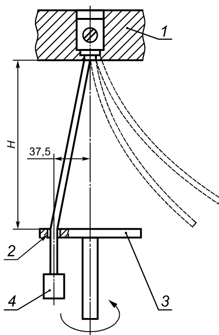
1 — фиксирующий узел; 2 — гильза; 3 — панель; 4 — груз
