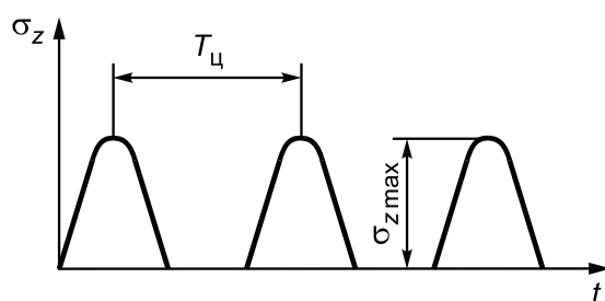
б) цикл напряжений
