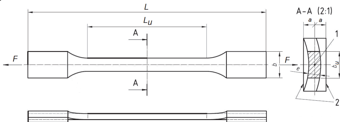
1 – центр тяжести поперечного сечения образца на измерительной базе; 2 – наращенные участки на концах образца; F – направление действия растягивающей силы; L – общая длина образца; L_u – длина измерительной базы; b – ширина образца в зажимах; 2a – толщина наращенной части концов образца; b_u – ширина образца на измерительной базе; e – толщина образца (стенки трубы)
