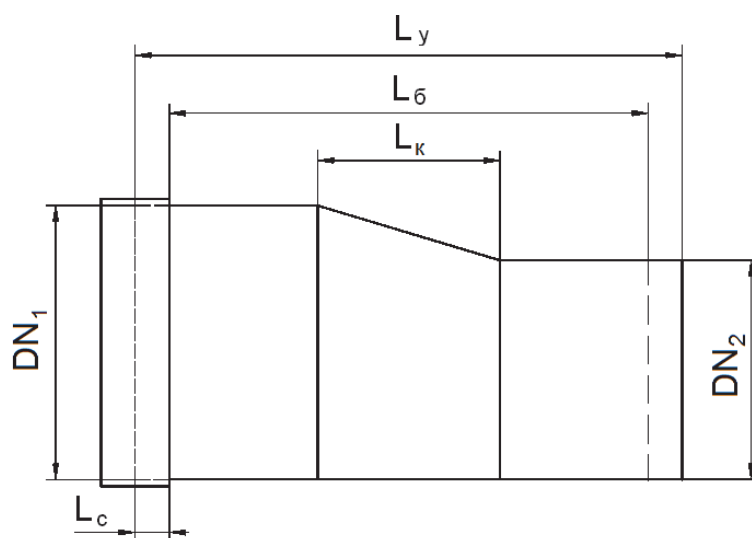
Рисунок А.5 – Эксцентрический переход
