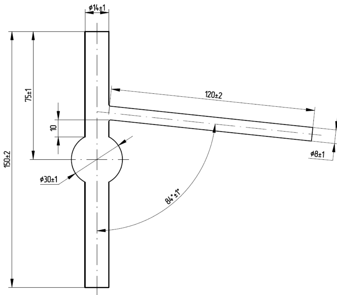
Рисунок 1 – Дефлегматор стеклянный одношариковый
