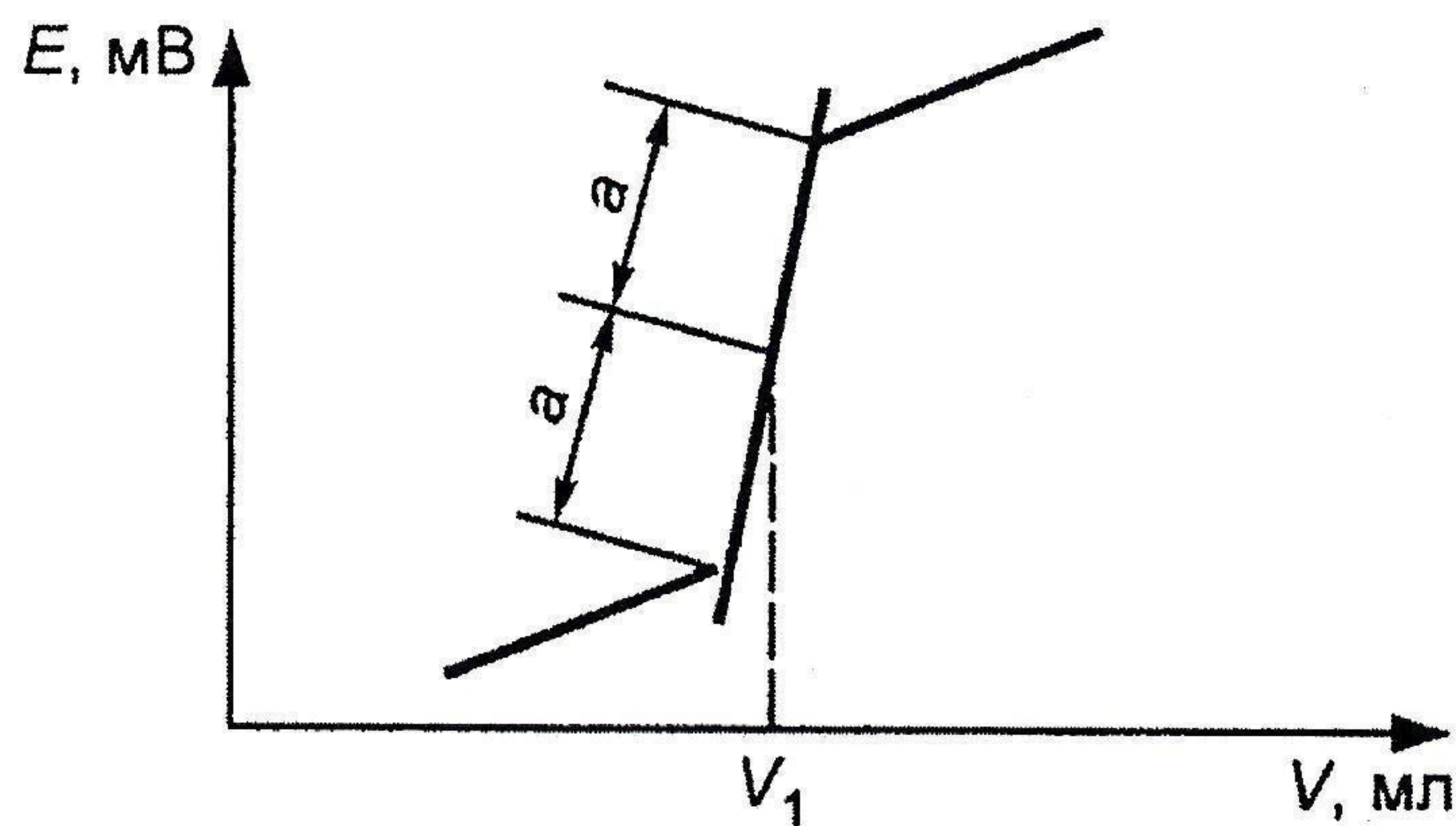
Рисунок 2 - Кривая титрования
