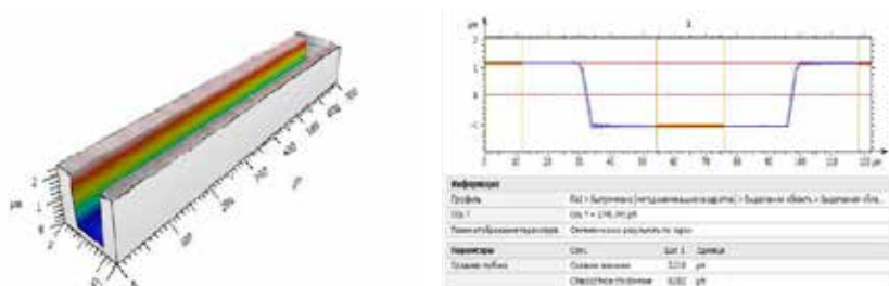
Рисунок 1.7 – Измеренная текстура поверхности одноштриховой меры ПРО-10 в 3D формате
