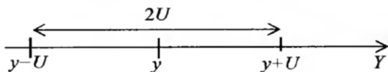
Рисунок 1.1 – К определению неопределенности измерения
