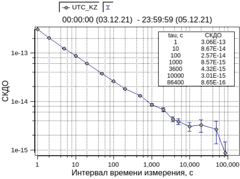
Рисунок 1.9 – Нестабильность частоты UTC(KZ)
