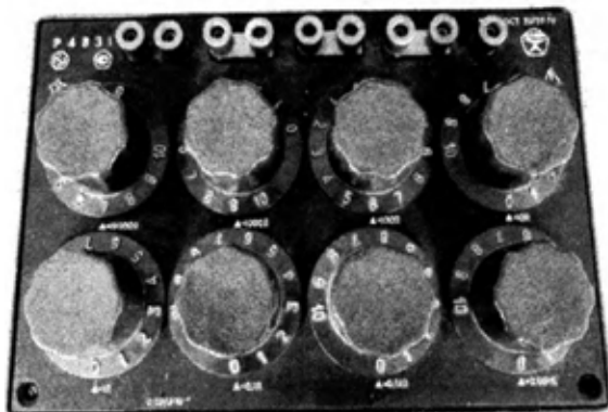
Рисунок 1.9 – Магазин сопротивлений класса точности 0,02/2 \cdot 10^{-6}
