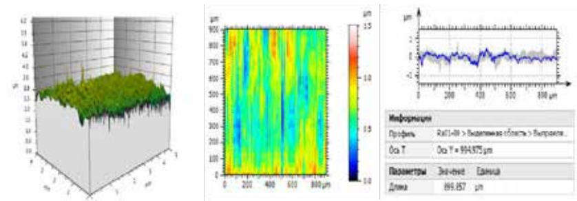
Рисунок 1.6 – Измеренная текстура поверхности меры ШП в 3D формате
