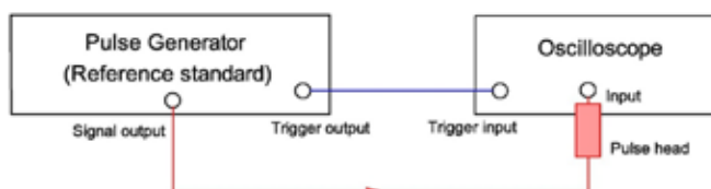
Рисунок 2.3 – Настройка для калибровки времени нарастания
