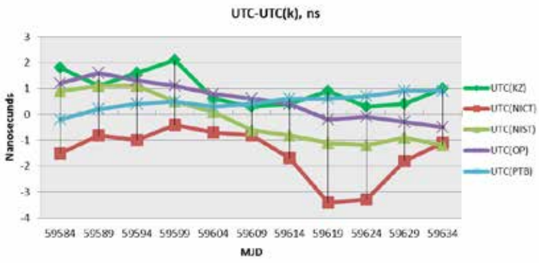
Рисунок 1.10 – Поведения национальной шкалы UTC(KZ) относительно UTC
