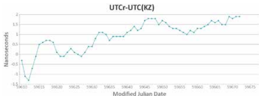
Рисунок 1.14 – Смещения шкал координированного времени относительно UTC
